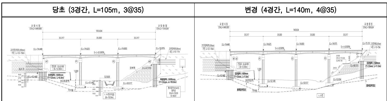
[그림] ㄴㄹ교 재설계 경간 변경 현황
